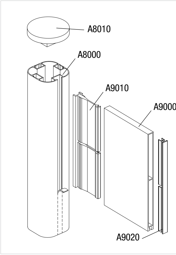
Profilo di chiusura in alluminio estruso per targhe bifacciali.
