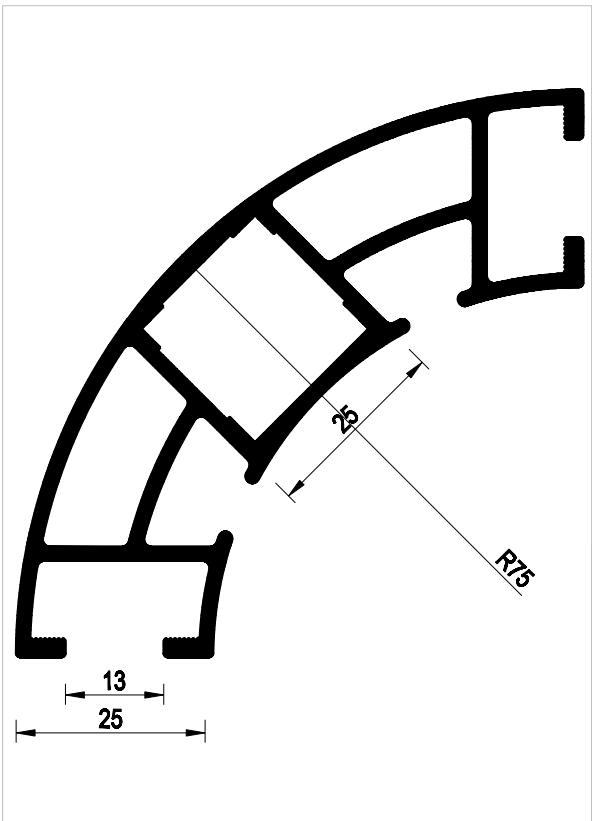
Profilo curvo in alluminio estruso a due vie a 90°. Lunghezza barre: 6000 mm.
