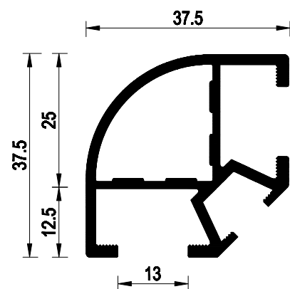
Profilo curvo in alluminio estruso a due vie a 90°. Lunghezza barre: 6000 mm.
