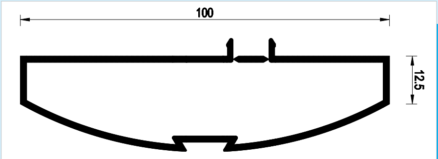
Profilo in alluminio estruso montante ornamentale curvo decentrato a scatto. Lunghezza barre: 5050 mm
