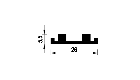
Rotaia inferiore 26x5,5. Lunghezza barre: 5000 mm.
