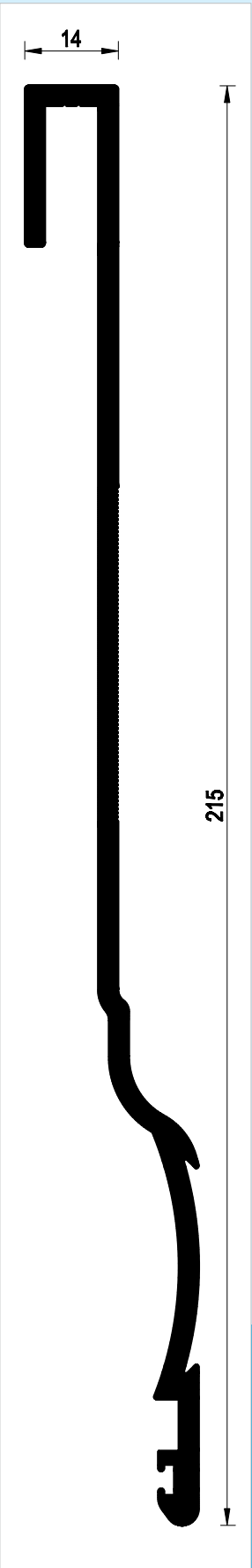
Profilo in alluminio estruso anta. Lunghezza barre: 5100 mm
