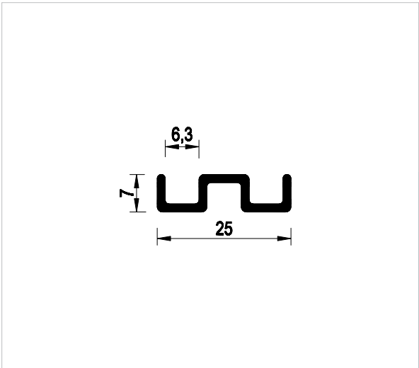
Guida inferiore 25x7. Lunghezza barre: 5000 mm.
