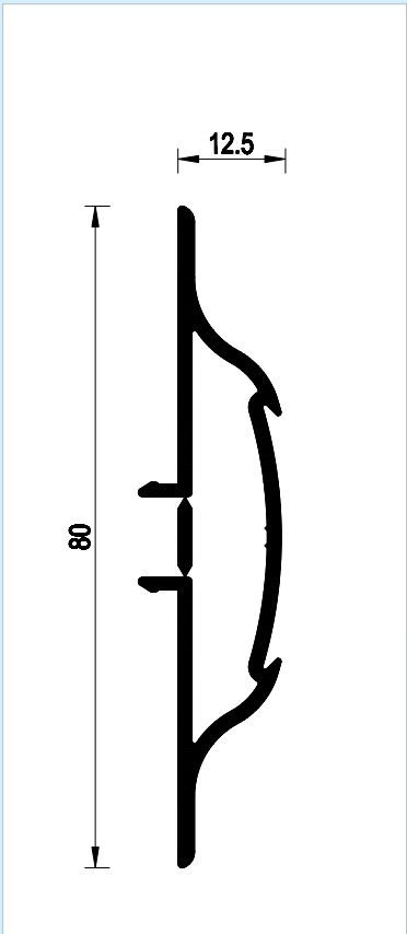
Profilo in alluminio traversa ornamentale curva a scatto. Lunghezza barre: 6000 mm.
