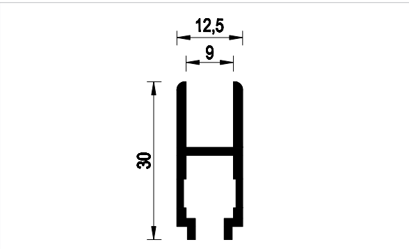
Per carrello di scorrimento 12,5x30. Lunghezza barre: 5000 mm.
