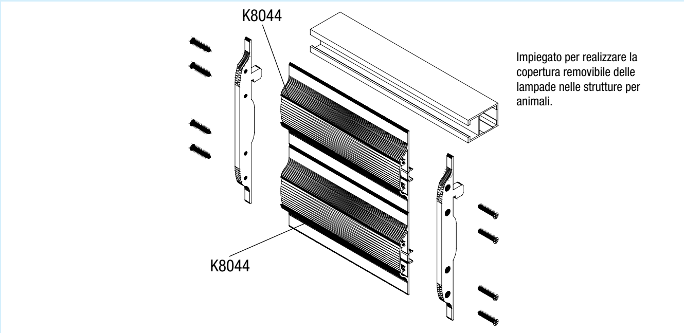
Kit per accoppiamento K8044 H: 180mm
