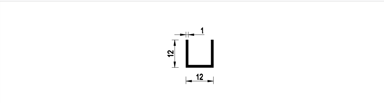
Profilo in alluminio estruso a "U" dimensione 12x12x1. Lunghezza barre: 6000 mm.
