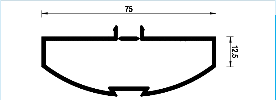
Profilo in alluminio estruso montante ornamentale curvo centrato a scatto. Lunghezza barre: 5050 mm
