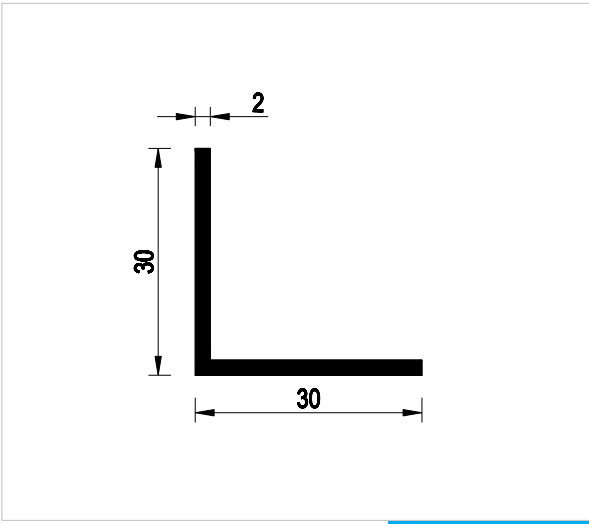
Profilo in alluminio estruso a "L" dimensione 30x30x2. Lunghezza barre: 6000 mm.
