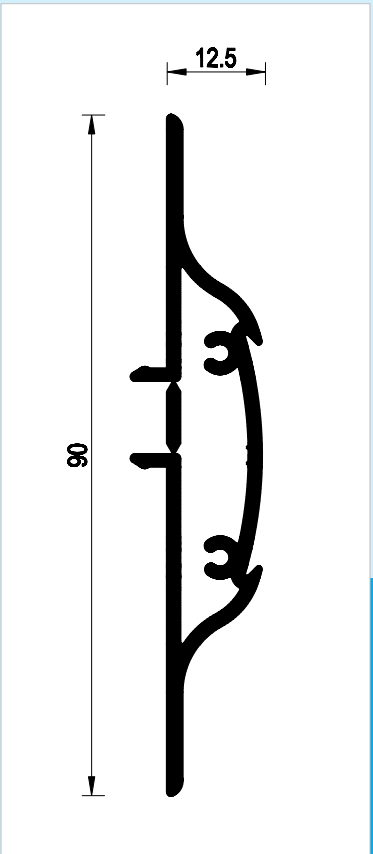
Profilo in alluminio traversa ornamentale maggiorato a scatto decentrato. Lunghezza barre: 6000 mm.
