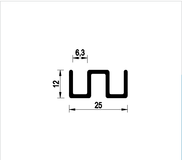
Guida superiore 25x12. Lunghezza barre: 5000 mm.
