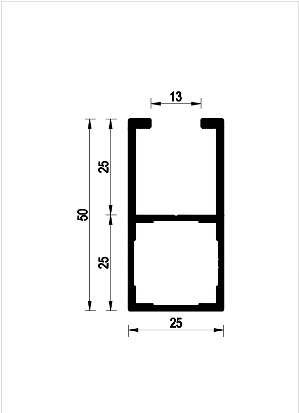
Profilo in alluminio estruso colonna - traversa a una via. Lunghezza barre: 6050 mm
