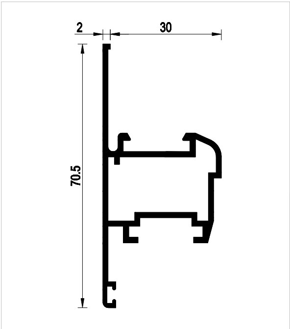
Profilo in alluminio estruso anta con fermavetro a scatto. Lunghezza barre: 6000 mm. A3700
