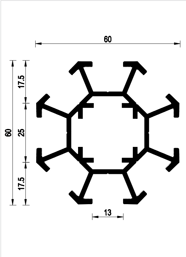
Profilo in alluminio estruso colonna a otto vie. Lunghezza barre: 5050 mm
