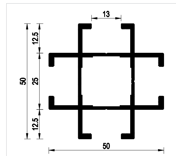
Profilo in alluminio estruso colonna - traversa a quattro vie. Lunghezza barre: 5050 mm
