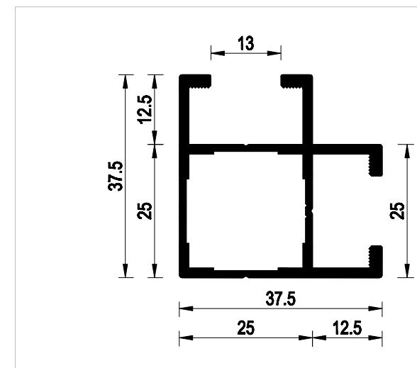
Profilo in alluminio estruso colonna - traversa a due vie a 90°. Lunghezza barre: 5050 mm
