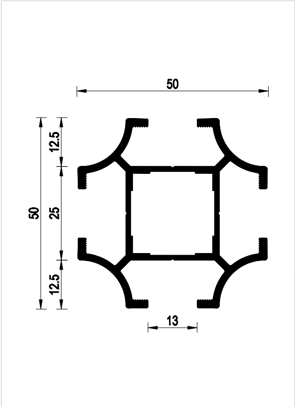
Profilo in alluminio estruso colonna a quattro vie. Lunghezza barre: 5050 mm
