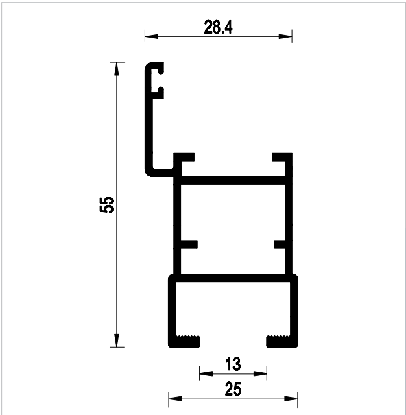
Profilo in alluminio estruso anta per vetro a infilare. Lunghezza barre: 6000 mm
