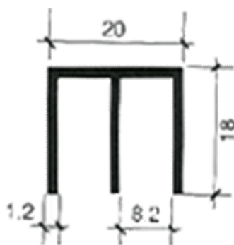
Perfil MT450
